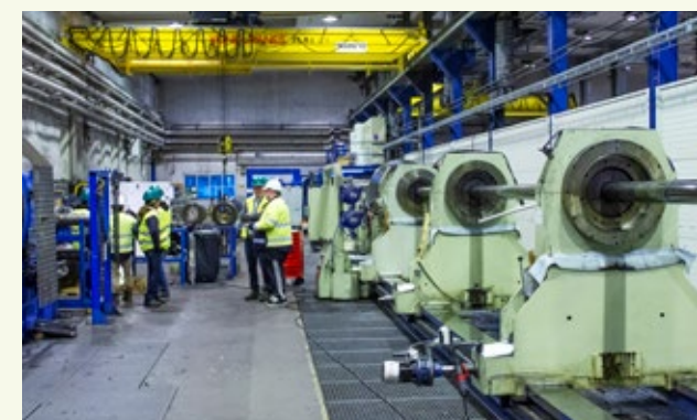
Borrmaskin på mekaniska verkstaden. Företaget investerade i utrustningen för tre år sedan för att kunna borra centrumhål i marina axlar upp till 22,5 meter.
